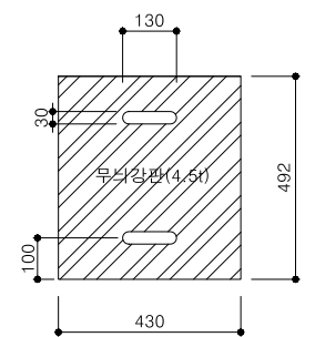
무늬강판 상세
